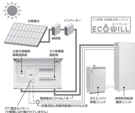
家庭用ガス発電・給湯暖房機+太陽光発電システム用電気系統接続概要図
