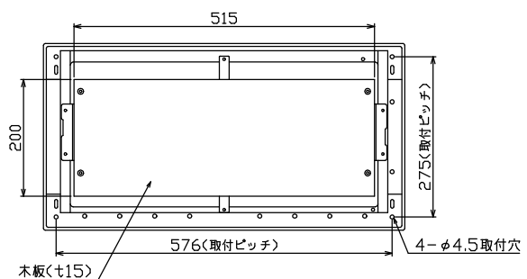
配線孔寸法図(//部開口)
