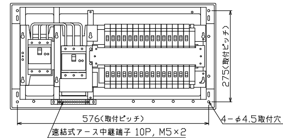
連結式アース中継端子 10P, M5×2
