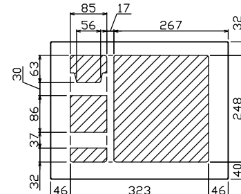
配線孔寸法図(//部開口)
