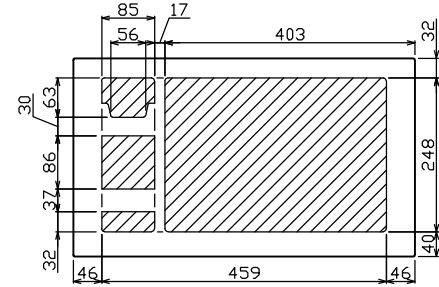
配線寸法図(//部開口)
