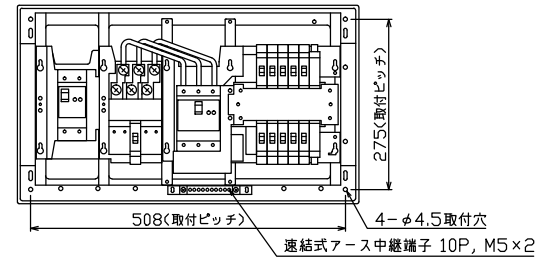
配線寸法図(//部開口)
