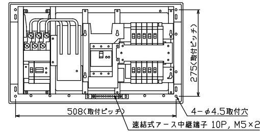
配線寸法図(斜線部開口)
