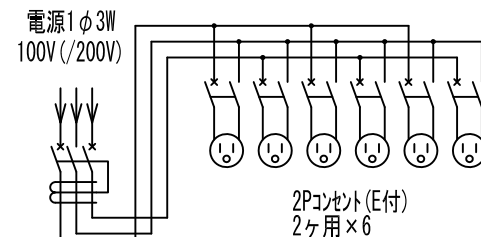
結線図
