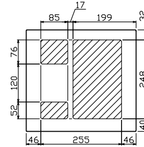
配線孔寸法図(斜線部開口)
