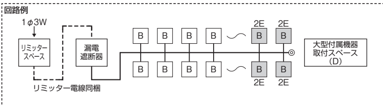
色:マンセル8GY9.7/0.2 リミッタースペース寸法 パールテクト(扉付) 大型付属機器取付スペース(D)付 175×178×64 タテ ヨコ フカサ
