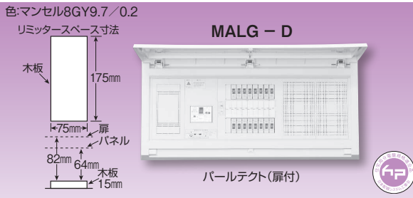
色:マンセル8GY9.7/0.2 リミッタースペース寸法 パールテクト(扉付) 大型付属機器取付スペース(D)付 175×178×64
