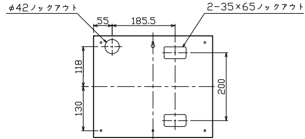
ケース底面ロックアウト図
