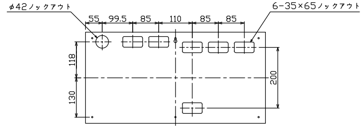
ケース底面ノックアウト図
