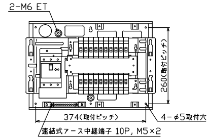
ケース底面ロックアウト図
