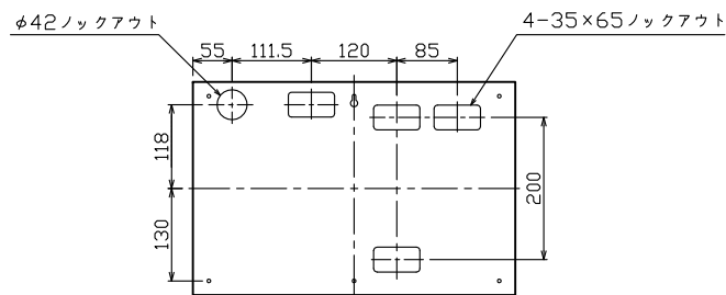
ケース底面ロックアウト図
