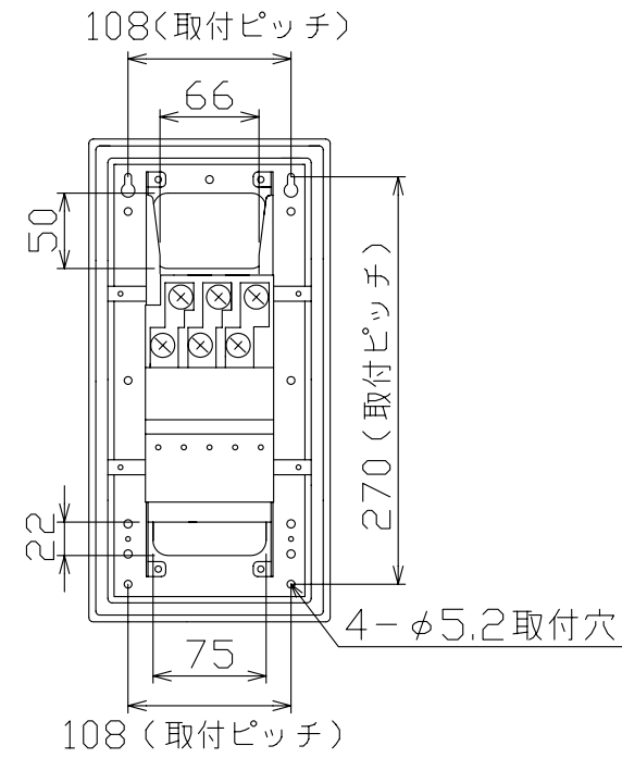
配線孔寸法図(////部開口)
