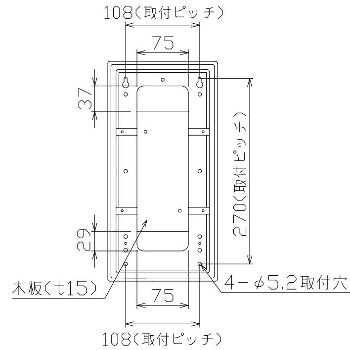
配線孔寸法図(////部開口)
